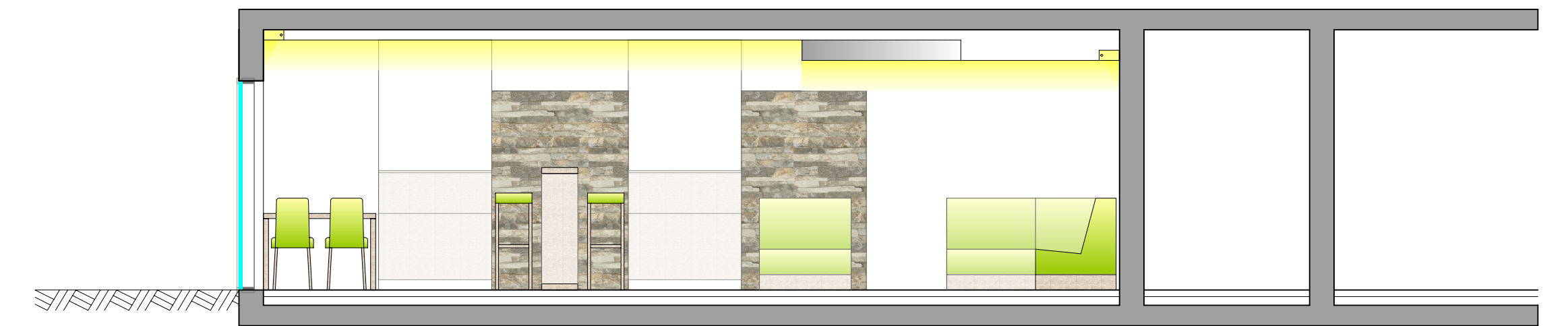
Schnitt B-B M.1:50
